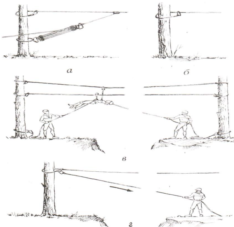
Технические приемы на навесной переправе:
